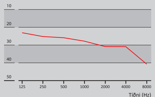
Meðaltalsdempun (dB) - Málmgreinanlegt sílikon
